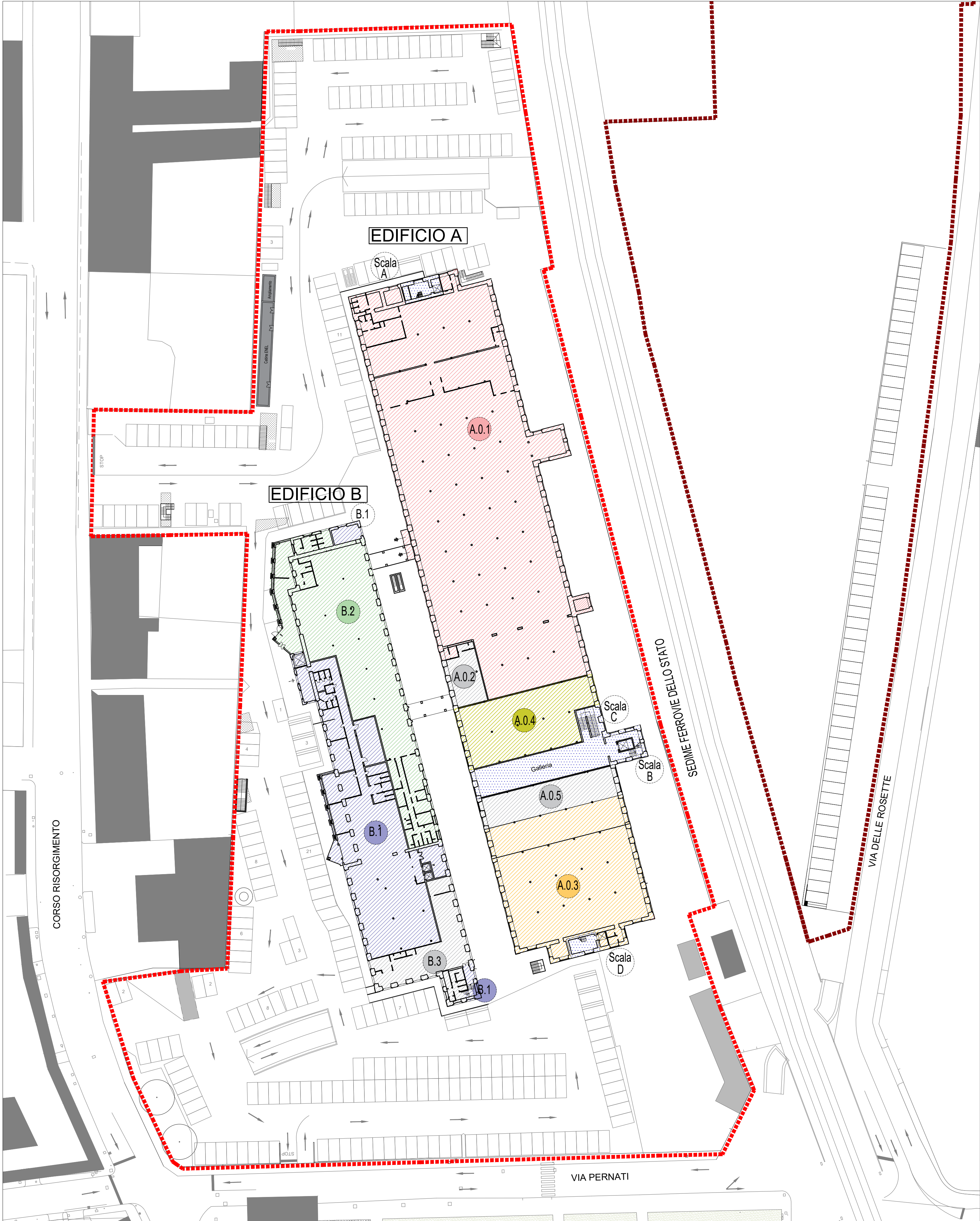
PLANIMETRIA PIANO TERRENO
